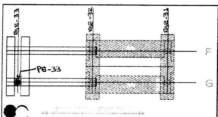
VISTA EN PLANTA DE LA UBICACIÓN DEL PILOTE OESTE (MAR)
