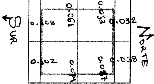
VISTA EN PLANTA DEL PILOTE ESTE (COSTA)
