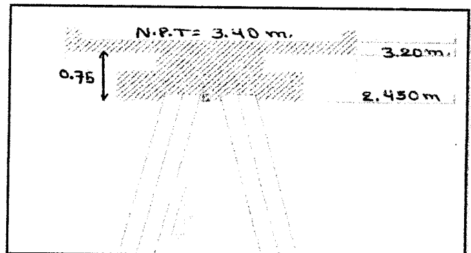
VISTA EN ELEVACION DEL PILOTE
